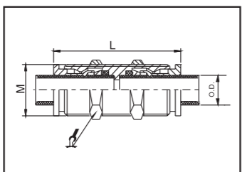
Вставной фитинг с резьбой и фиксирующей гайкой
