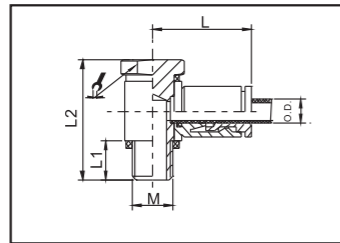
Вставной с прямым углом фитинг для конечного регулируемого соединения
