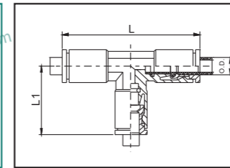
Вставной тройник-фитинг
